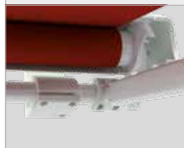
Armbefestigung am Tragrohr
