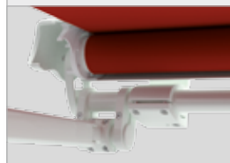
Versetzter Gelenkarm am stabilen Tragrohrabschnitt befestigt
